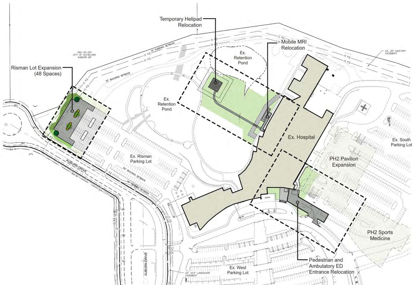
Enabling Diagram - Site Plan
