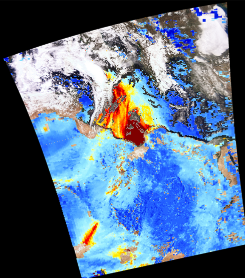
Aerosol Optical Depth 0.55 \mu\text{m} 0.00 0.25 0.50 0.75 1.00
