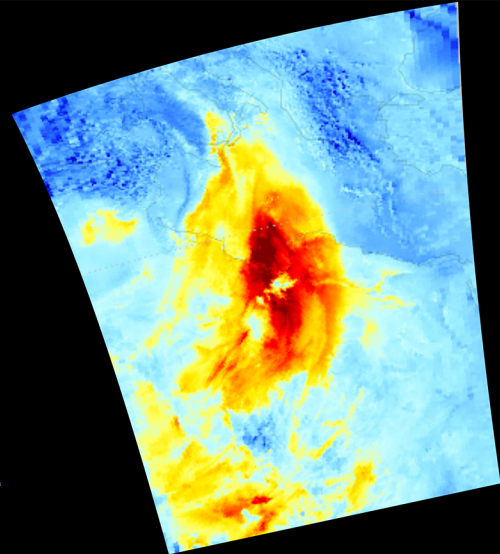
NUV Aerosol Index (UVAI) -1.0 0.2 1.4 2.6 3.8 5.0
